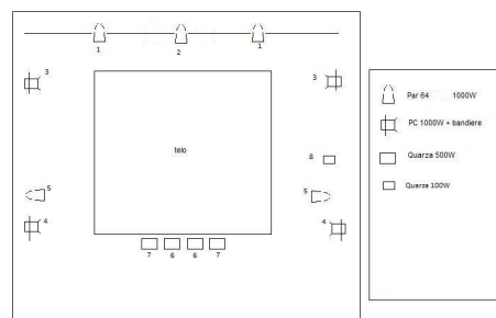
L'ISOLA - pianta luci -
